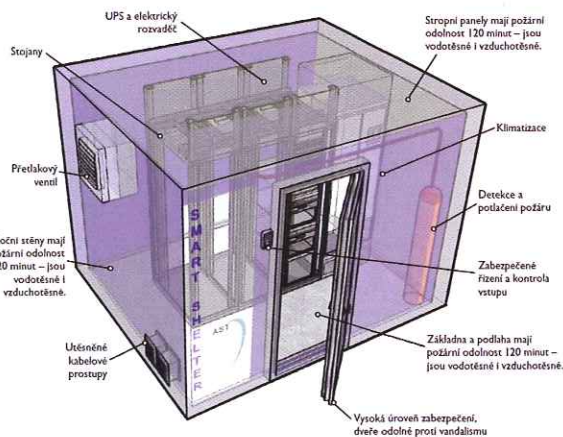
Klíčové prvky datové komory AST Smart Shelter
