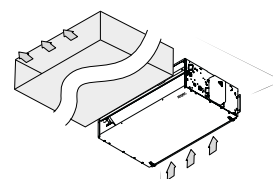
Mezistropní montáž s připojením k VZT potrubí
